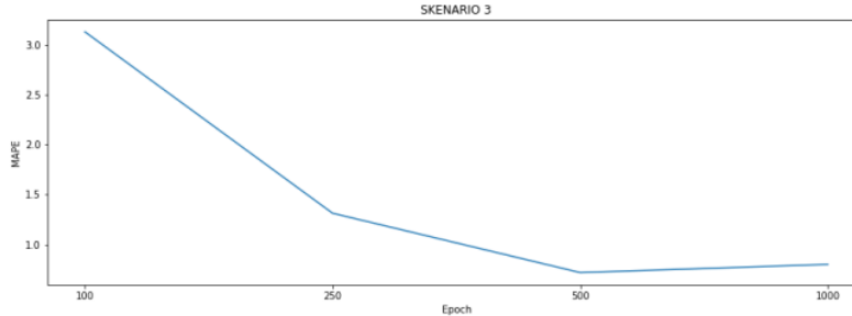
Gambar 9. Grafik skenario 3 penentuan epoch
