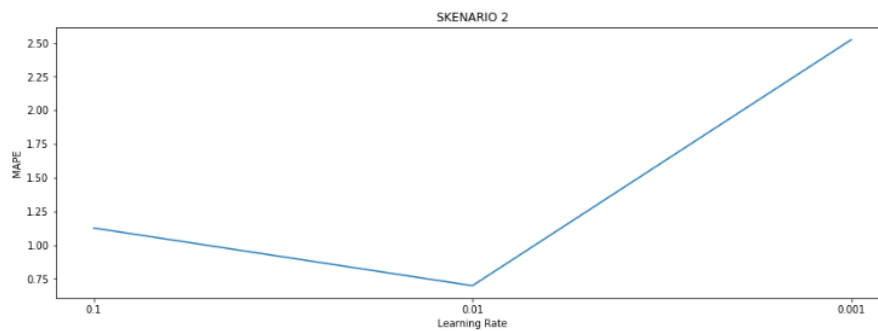
Gambar 8. Grafik skenario 2 pada learning rate 0,1, 0,01, dan 0,001
