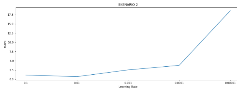
Gambar 8. Grafik skenario 2 penentuan learning rate
