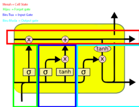
Gambar 2. Arsitektur LSTM
