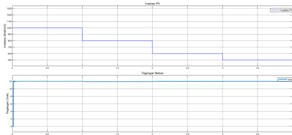
Gambar 9 Hasil Simulasi Irradiasi berfluktuasi Menggunakan Kontrol Tegangan.
