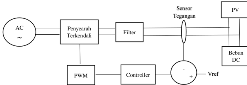
Gambar 1 Layout Jaringan Listrik DC
