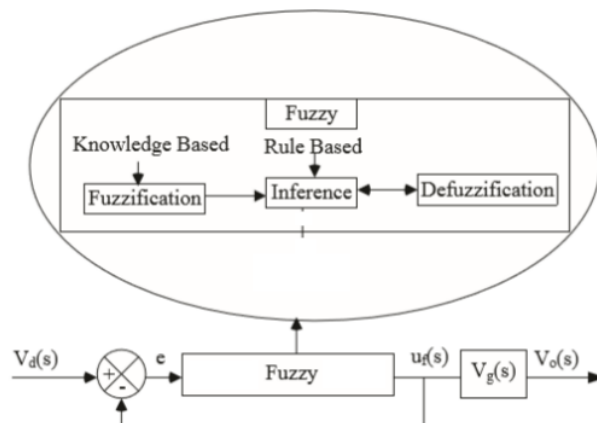
Gambar 2 Diagram Blok Sistem Kontrol Tegangan Menggunakan Fuzzy
