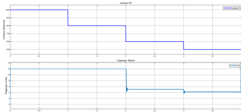
Gambar 8 Hasil Simulasi Irradiasi berfluktuasi Tanpa Kontrol Tegangan.
