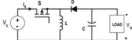
Gambar 3. Rangkaian Buck Boost Converter
