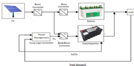
Gambar 1. Konfigurasi Jaringan DC Microgrid
