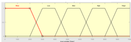
Gambar 5. Fungsi Keanggotaan Masukan Pdem
