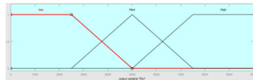
Gambar 6. Fungsi Keanggotaan Keluaran Psc
