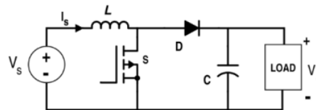
Gambar 2. Rangkaian Boost Converter
