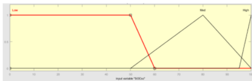
Gambar 4. Fungsi Keanggotaan Masukan SoC SC
