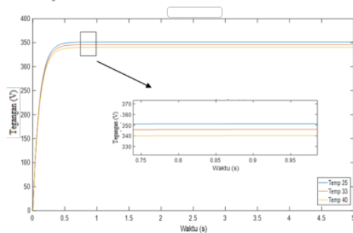
Gambar 9. Tegangan PV saat T (beda) Ir (sama)
