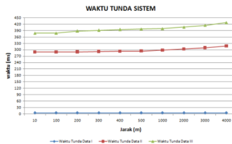
Gambar 15. Grafik Waktu Tunda Sistem
