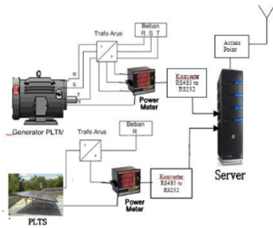
Gambar 1. Diagram Blok Alat
