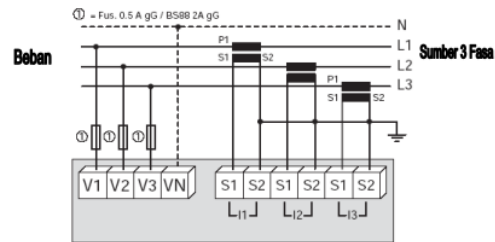
Gambar 3. Diagram pengawatan powermeter dengan beban dan sumber tegangan
