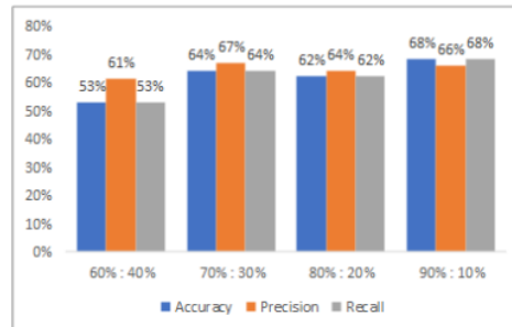
Gambar 3. Grafik hasil pengujian naïve bayes
