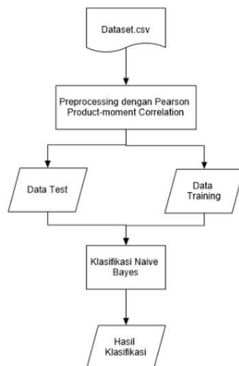
Gambar 1. Skema implementasi dan pengujian
