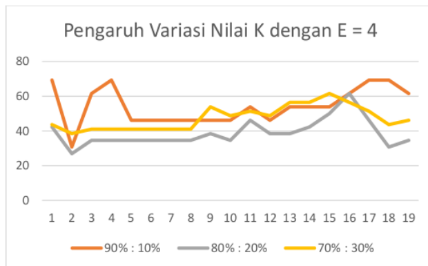
Gambar 8. Grafik Perubahan Nilai k dengan Nilai e = 4
