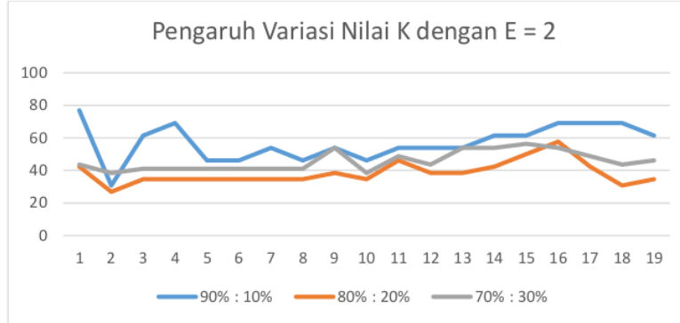
Gambar 7. Grafik Perubahan Nilai k dengan Nilai e = 2
