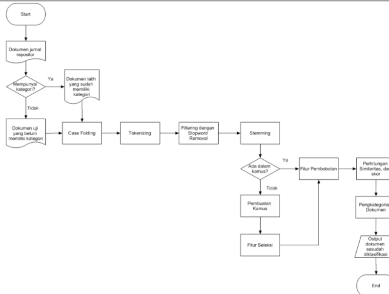
Gambar 1. Alur Tools Klasifikasi Repositor Jurnal Teknik Informatika UMM
