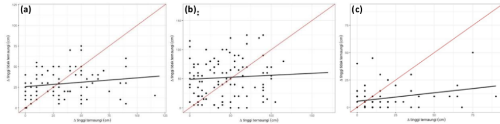
Gambar 5. Scatter plot antara tinggi ternaung dan tidak ternaung pada jenis (a) gayam, (b) puspa, dan (c) salam antara tinggi ternaungi (sumbu horizontal) vs tinggi tidak ternaung (sumbu vertikal). Garis hitam adalah garis regresi. Garis diagonal merah adalah garis 1:1. Setiap titik mewakili jenis tanaman.
