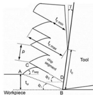
Gambar 5. Bentuk Geram bergerigi
