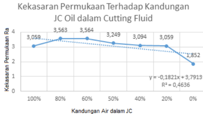
Gambar 2. Grafik Kekasaran Permukaan Terhadap Kandungan JC Oil dalam Cutting Fluid
