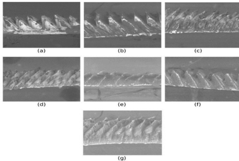
Gambar 4. Hasil foto mikro geram dari beberapa variasi : (a) geram dari kandungan JC 100%; (b) geram dari kandungan 80% JC + 20% air; (c) geram dari kandungan 60% JC + 40% air; (d) geram dari kandungan 50% JC + 50% air (e) geram dari kandungan 40% JC + 60% air; (f) geram dari kandungan 20% JC + 80% air; (g) geram dari kandungan air 100%.
