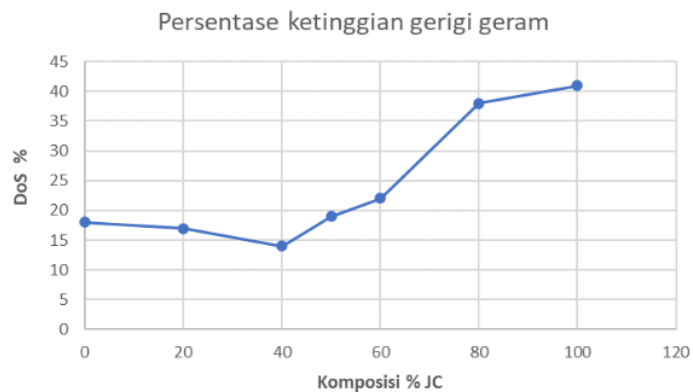
Gambar 7. Hasil perhitungan DoS gerigi geram
