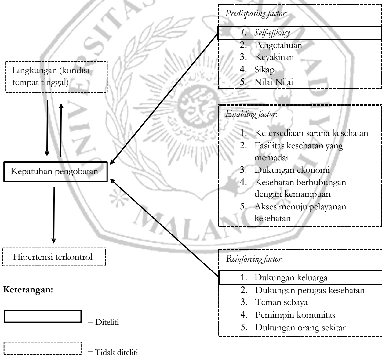
Gambar 3.1 Kerangka Konsep
