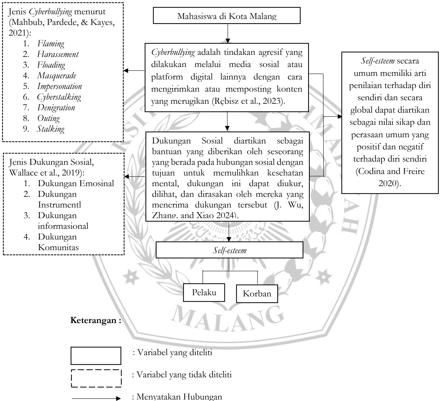
Gambar 3.1 Kerangka Konsep
