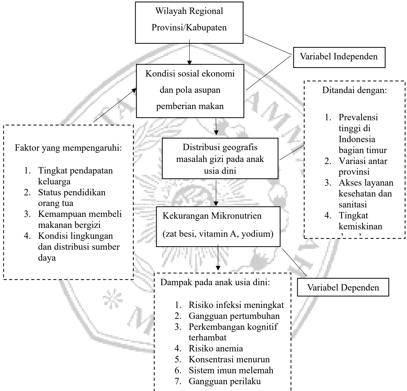
Gambar 3. 1 Kerangka Konsep
