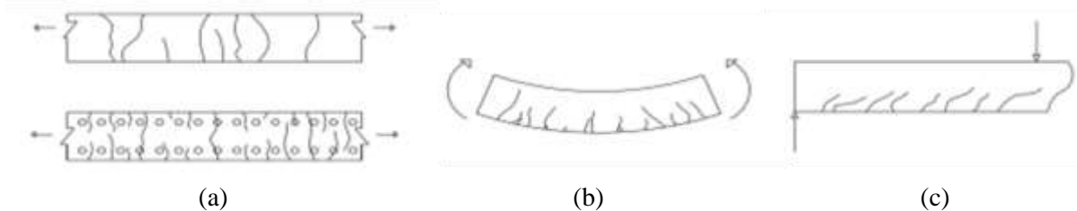
Gambar. 2. (a) Pola retak beton bertulang akibat gaya tarik, (b) Pola retak beton bertulang akibat momen, (c) Pola retak beton bertulang akibat geser. (Nawy, E.G 1998).
