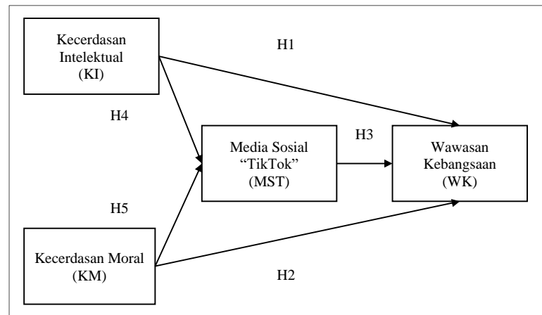
Gambar 2.1 Kerangka Teori
