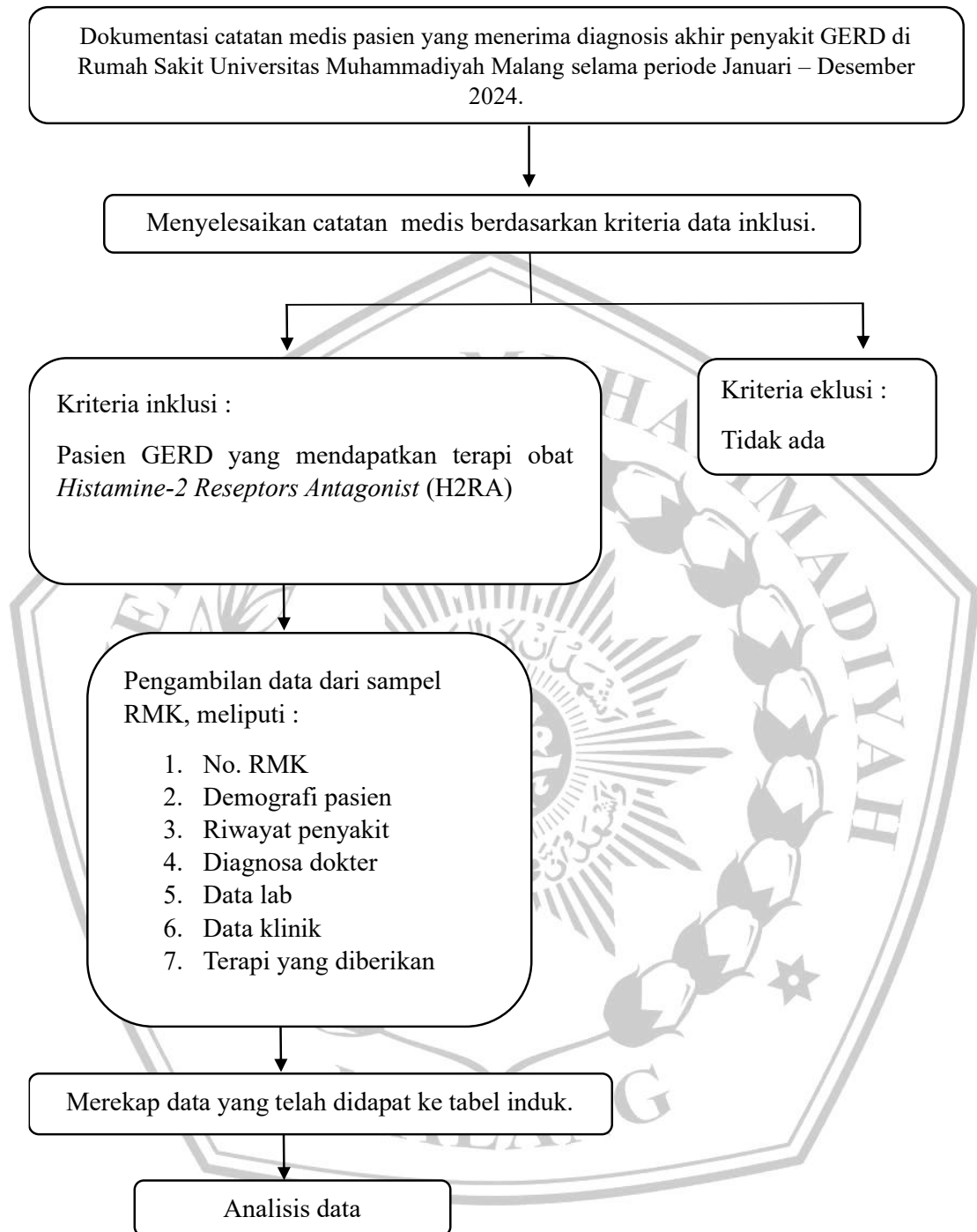
Gambar 3. 2 Kerangka Operasional
