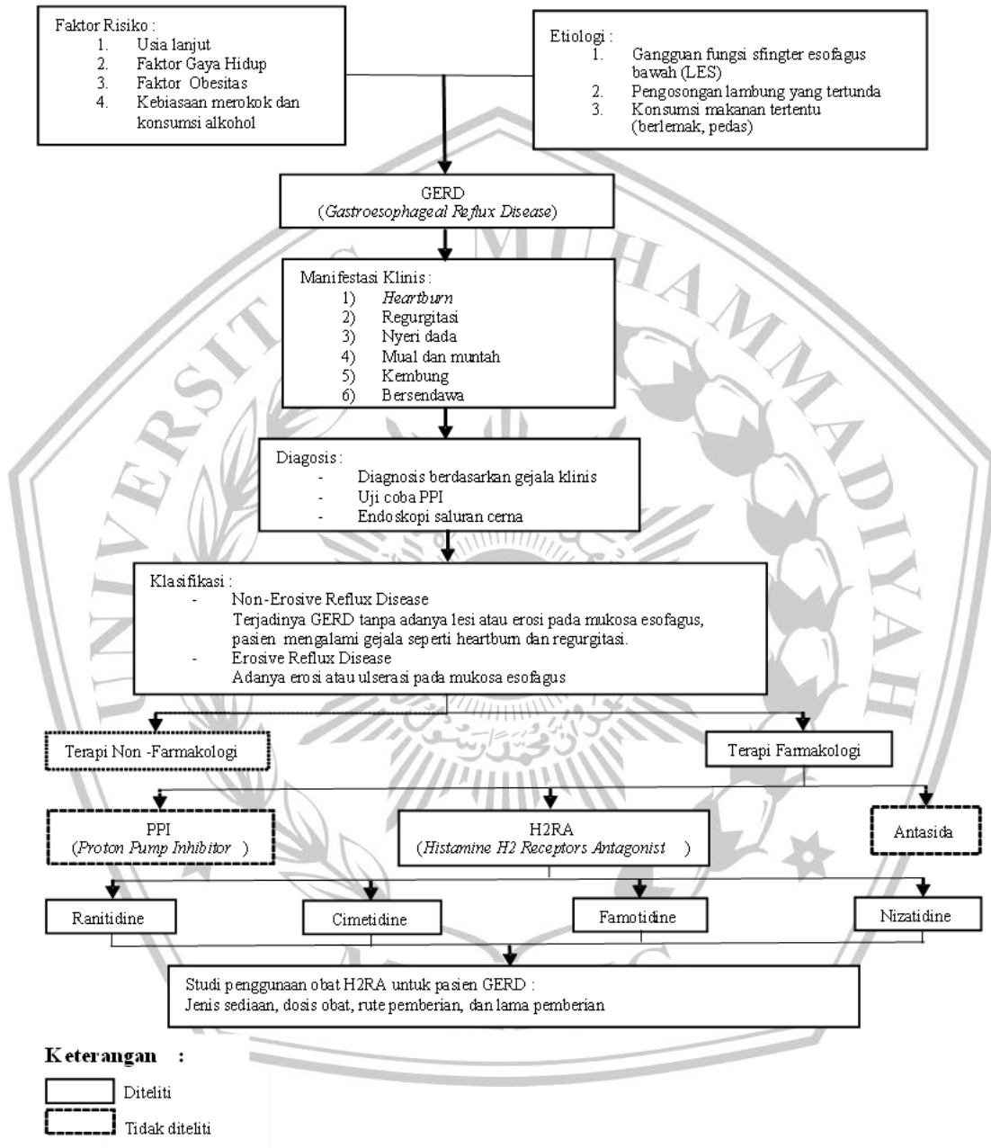
Gambar 3. 1 Kerangka Konseptual
