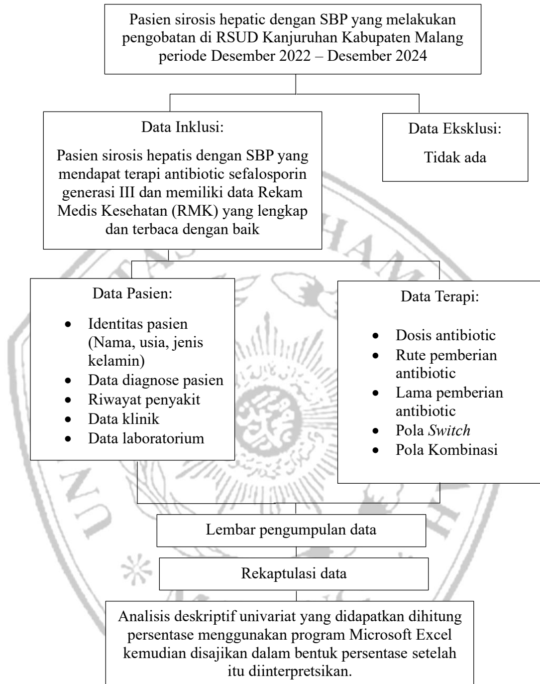
Gambar 3.2 Kerangka Operasional
