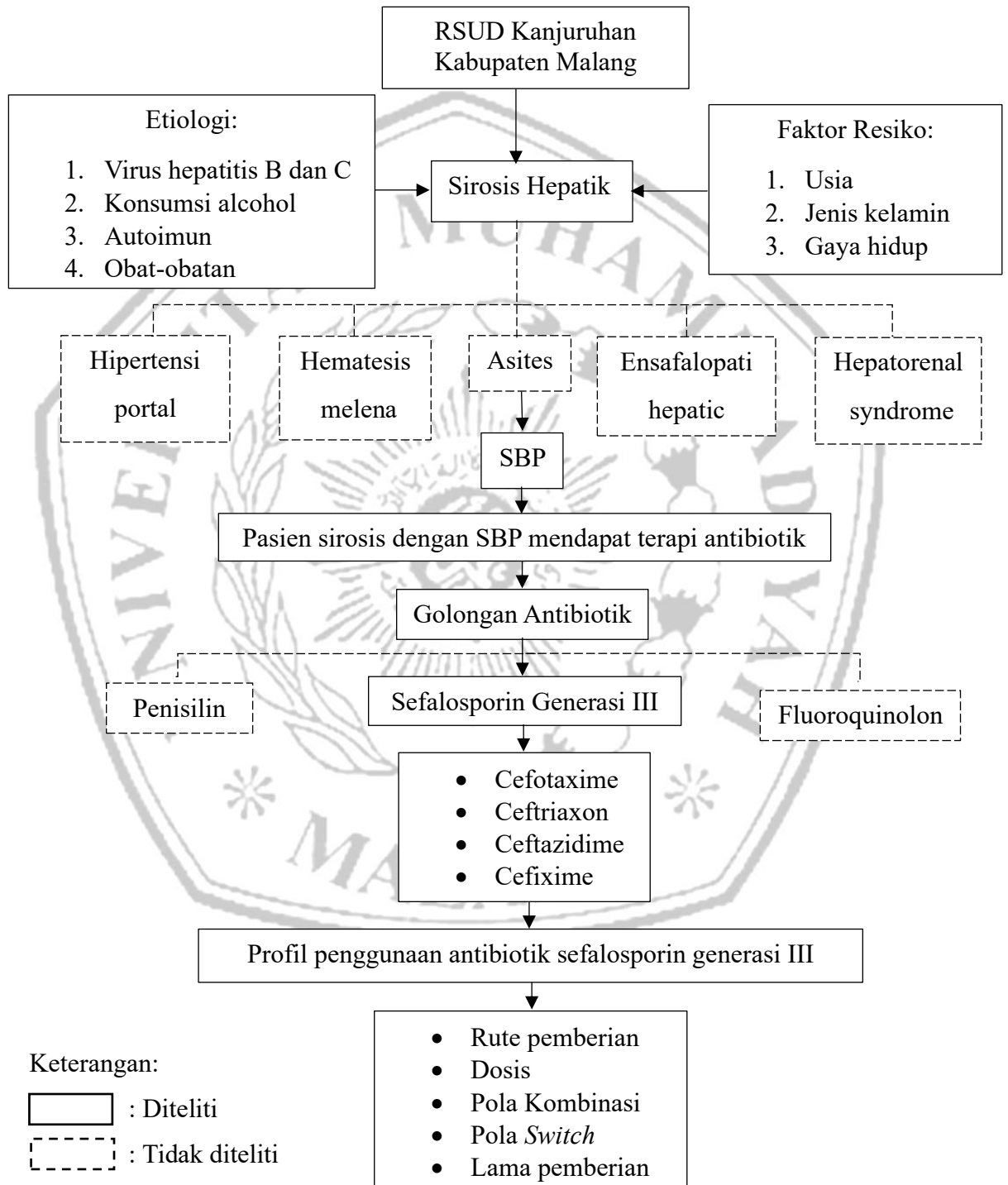
Gambar 3.1 Kerangka Konseptual
