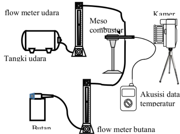
Gambar 1 Susunan instalasi penelitian untuk pembakar skala meso dengan bahan bakar cair
