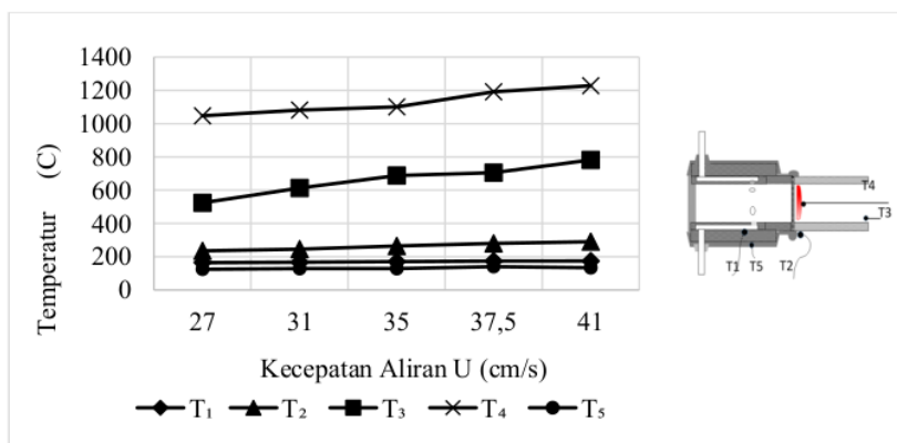
Gambar 6 Distribusi temperatur nyala butana pada \phi=1.4 pembakar skala meso SS.
