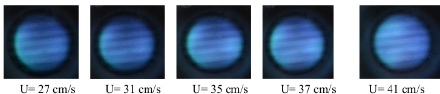
Gambar 5 Nyala butana pada rasio ekuivalen \phi = 0,75
