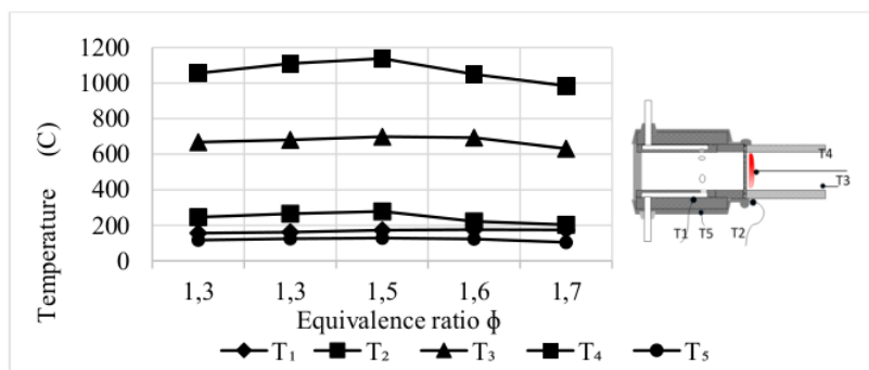
Gambar 7 Distribusi temperatur nyala butana pada U = 35 cm/s pembakar skala meso ss
