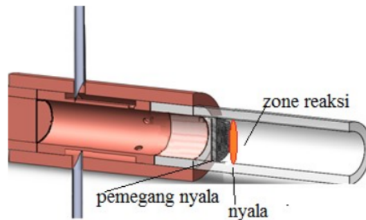
Gambar 2 Pembakar skala meso tipe A
