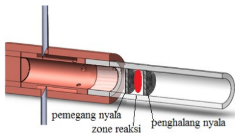
Gambar 3 Pembakar skala meso tipe B
