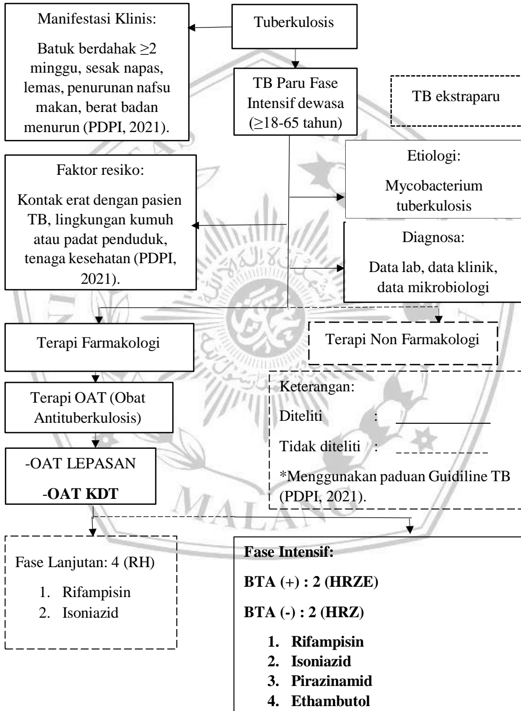
Gambar 3.1 Kerangka Konseptual
