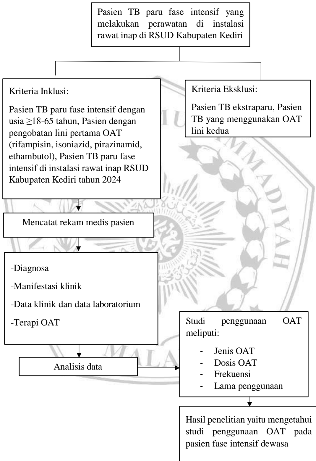
Gambar 3.2 Kerangka Operasional
