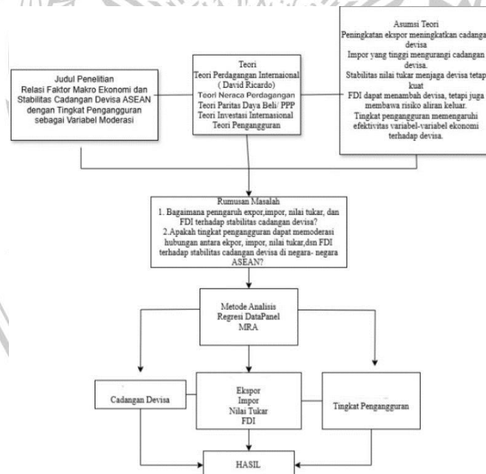
Gambar 2.1 Kerangka Pikir
