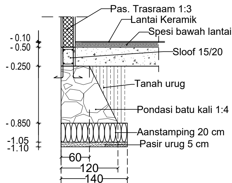
DETAIL PONDASI B SKALA ; 1 : 25
