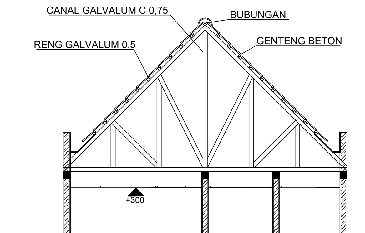
DETAIL POTONGAN KUDA KUDA AA SKALA ; 1 : 50
