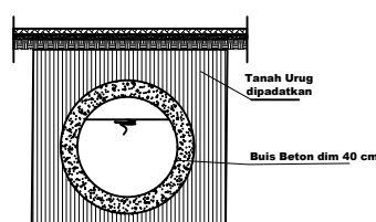
SALURAN DRAINASE
