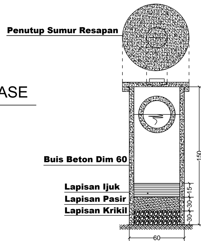
SUMUR RESAPAN
