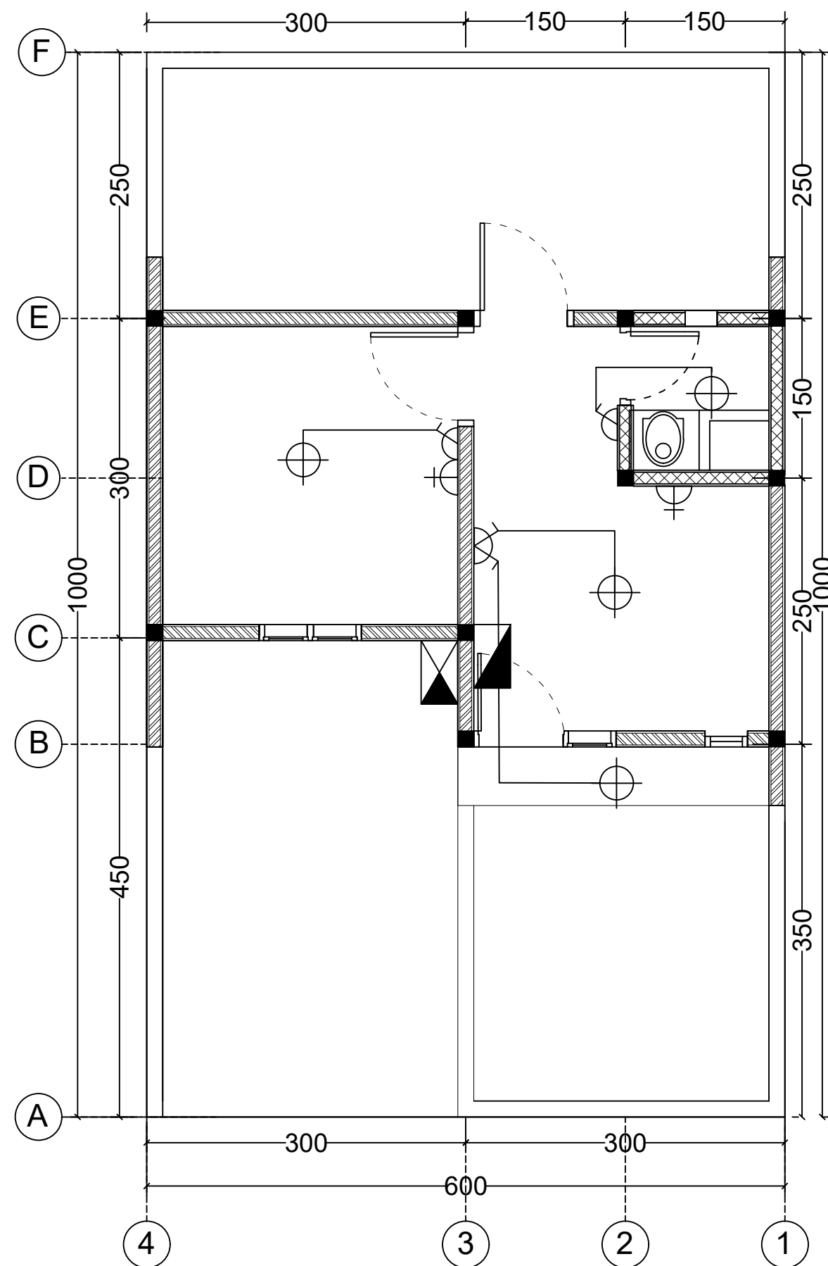
RENCANA TITIK LAMPU DAN STOP KONTAK SKALA : 1 : 50
