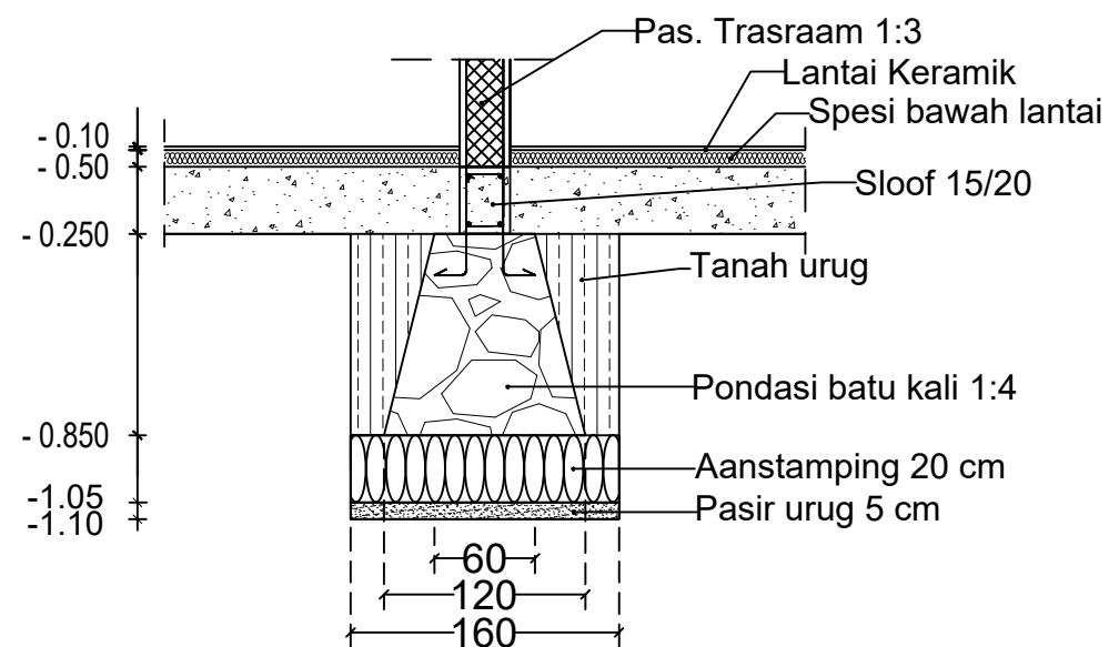
DETAIL PONDASI A SKALA ; 1 : 25
