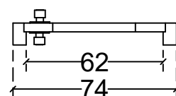
DETAIL J 02 SKALA ; 1 : 25
