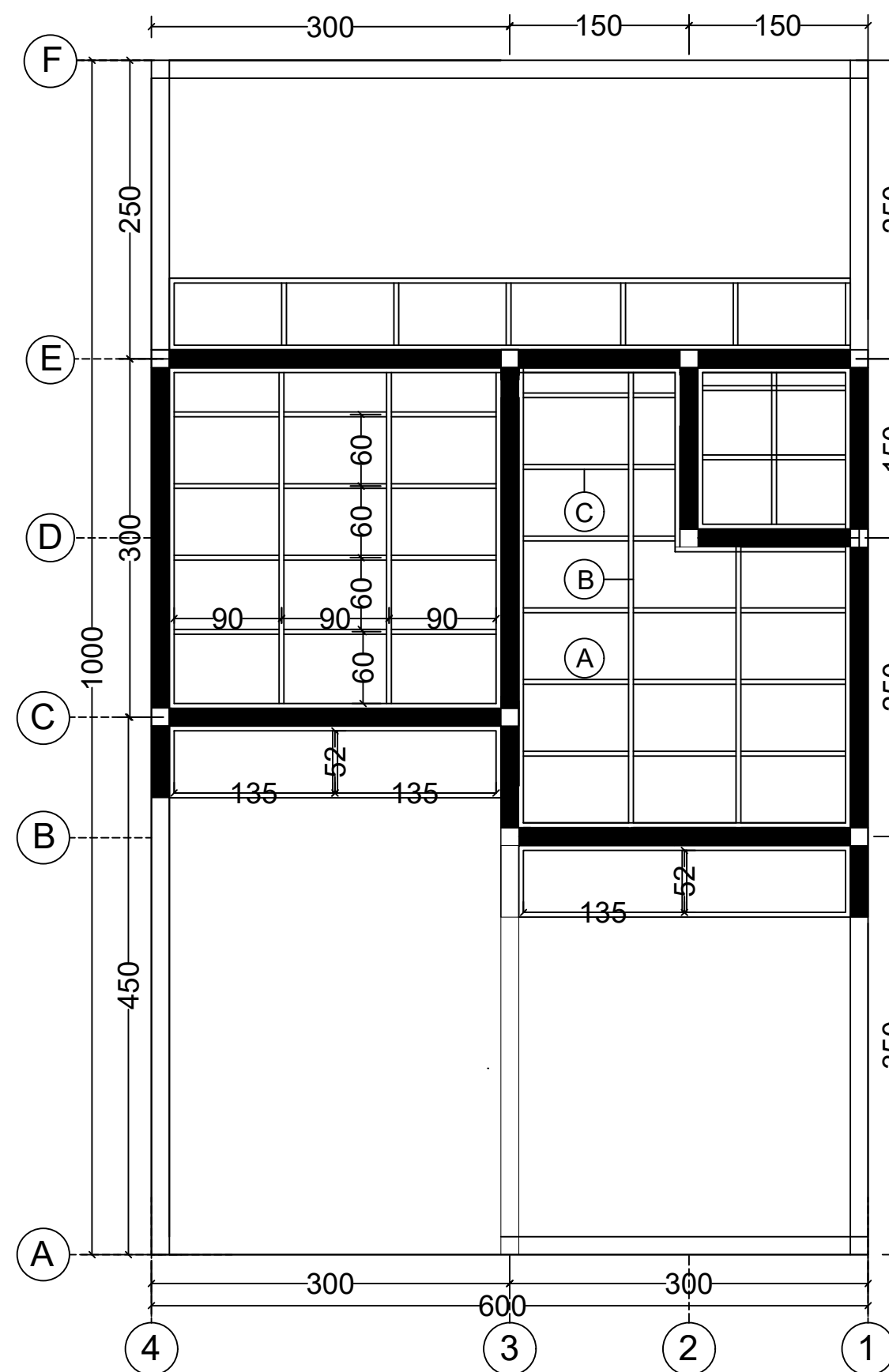
RENCANA PLAFOND SKALA : 1 : 50
