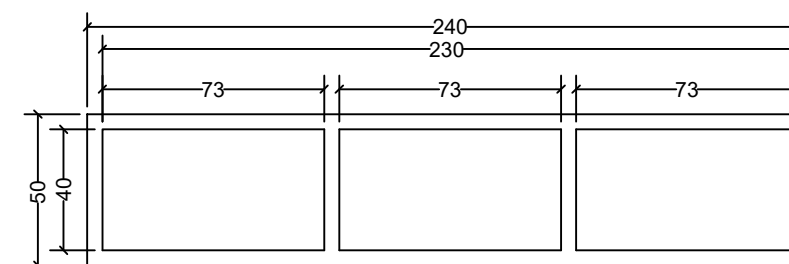
DETAIL VENTILASI KACA SKALA ; 1 : 25
