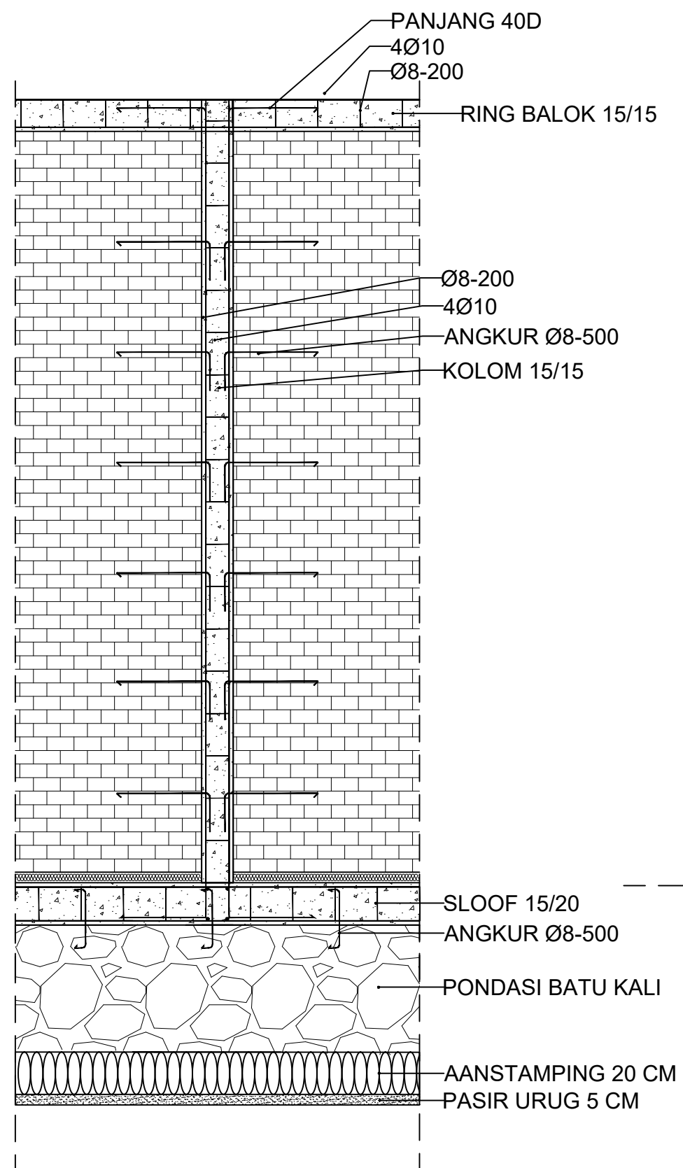
PEMBESIAN PONDASI SLOOF KOLOM & BALOK SKALA ; 1 : 25
