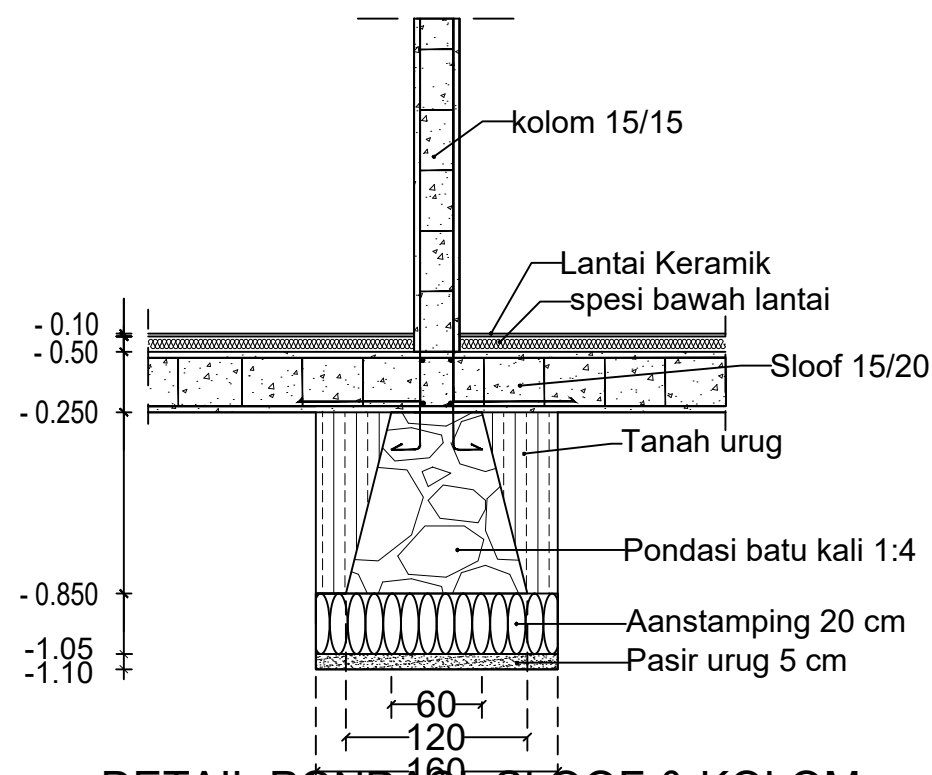
DETAIL PONDASI, SLOOF & KOLOM SKALA ; 1 : 25
