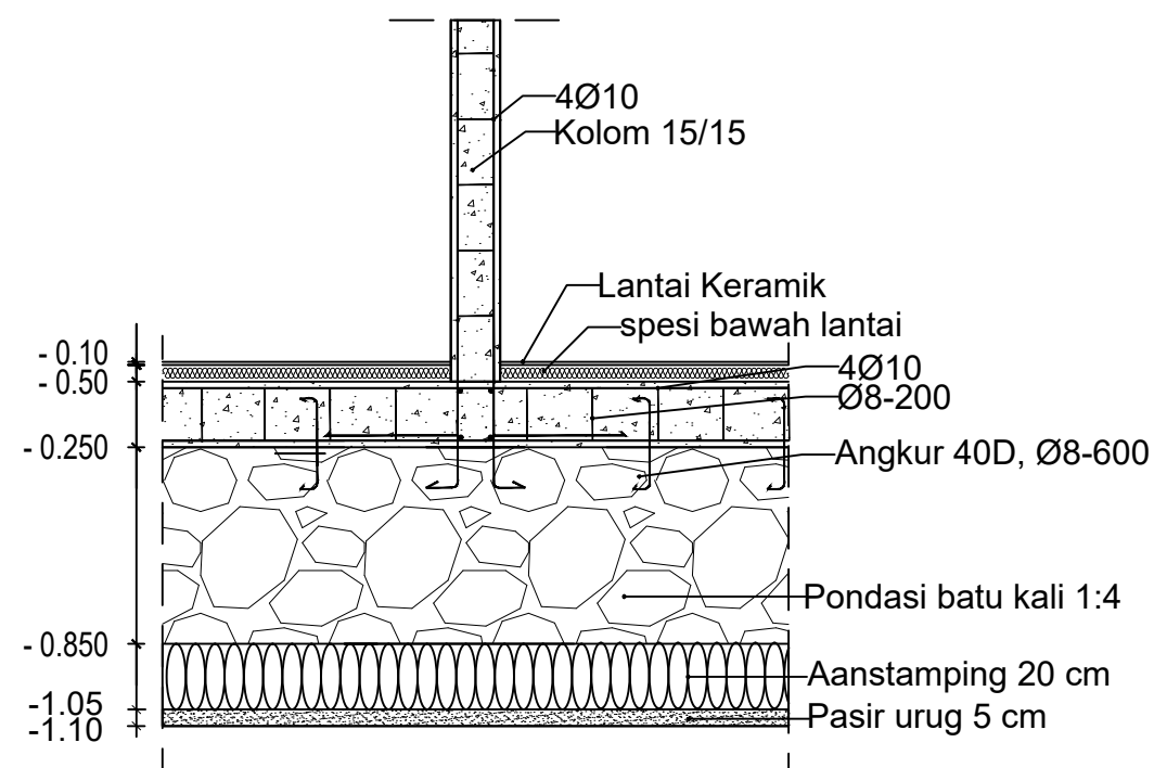
PEMBESIAN KOLOM, SLOOF & PONDASI SKALA ; 1 : 25
