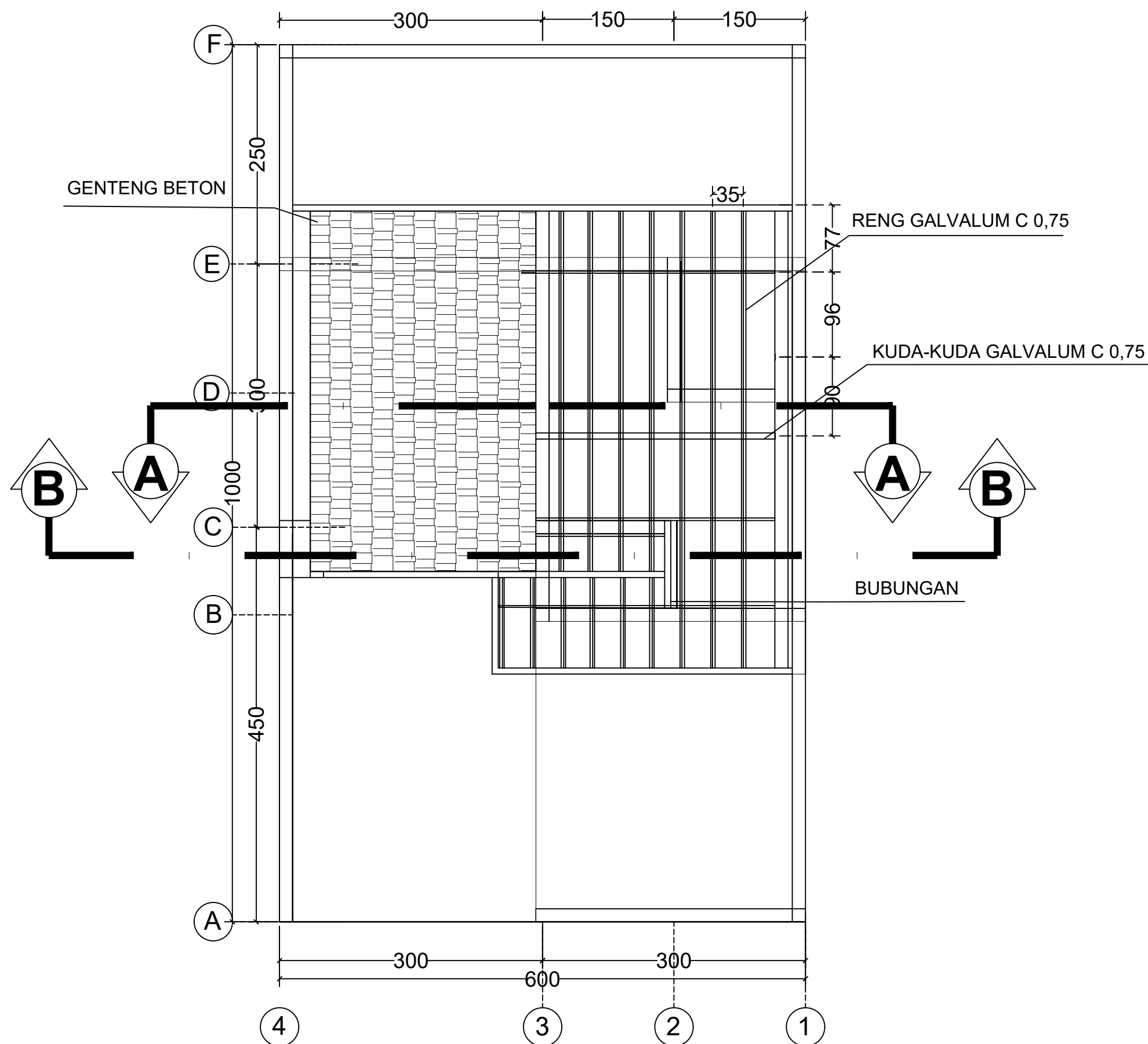
RENCANA ATAP SKALA ; 1 : 50
