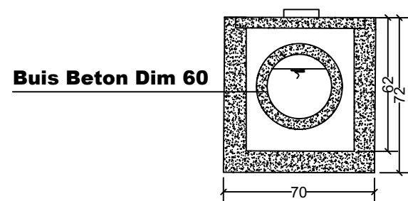
BAK KONTROL DRAINASE
