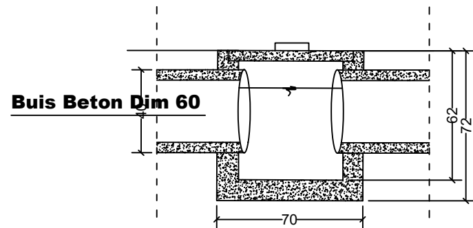
BAK KONTROL DRAINASE
