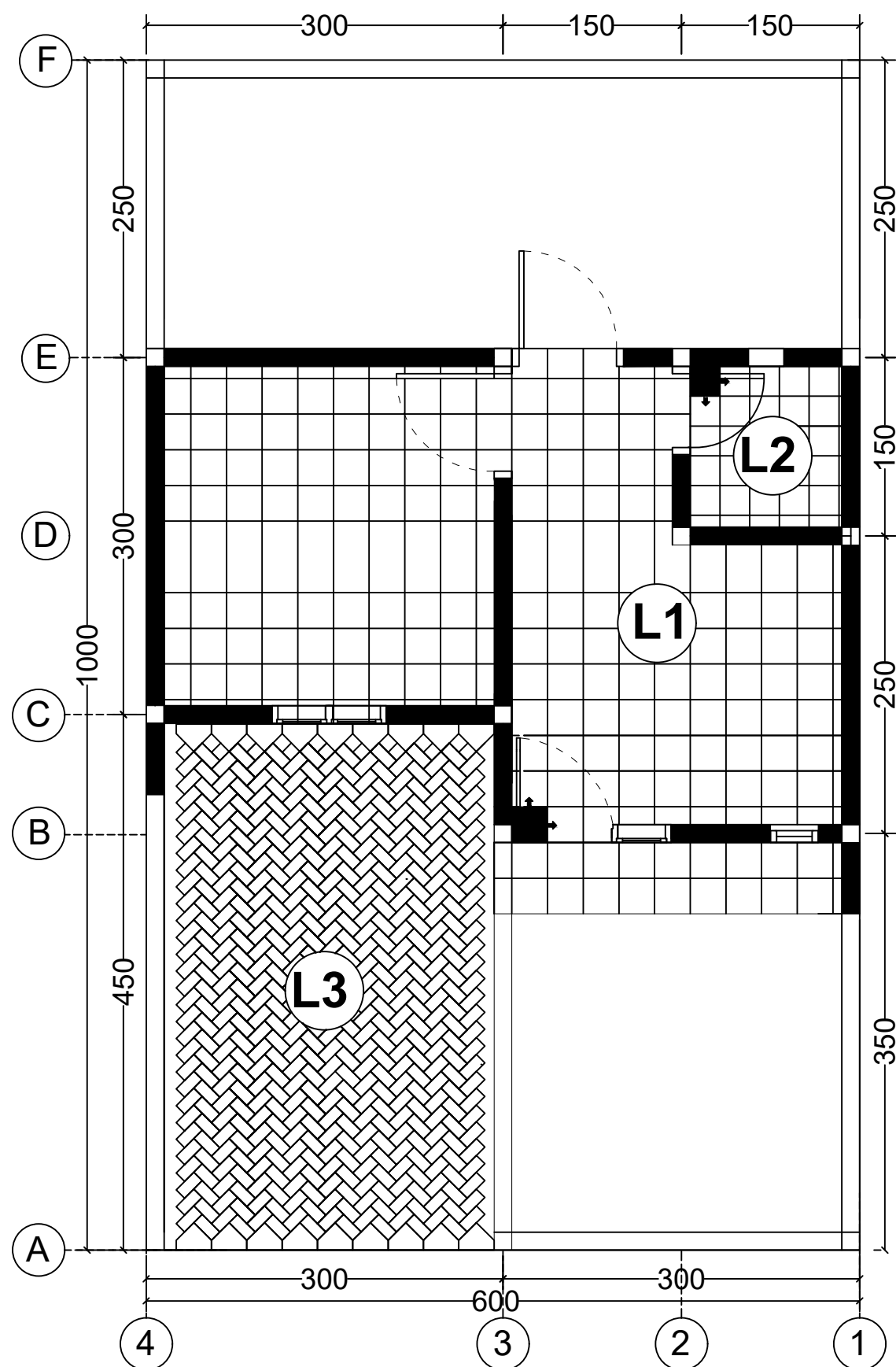
RENCANA LANTAI SKALA : 1 : 50
