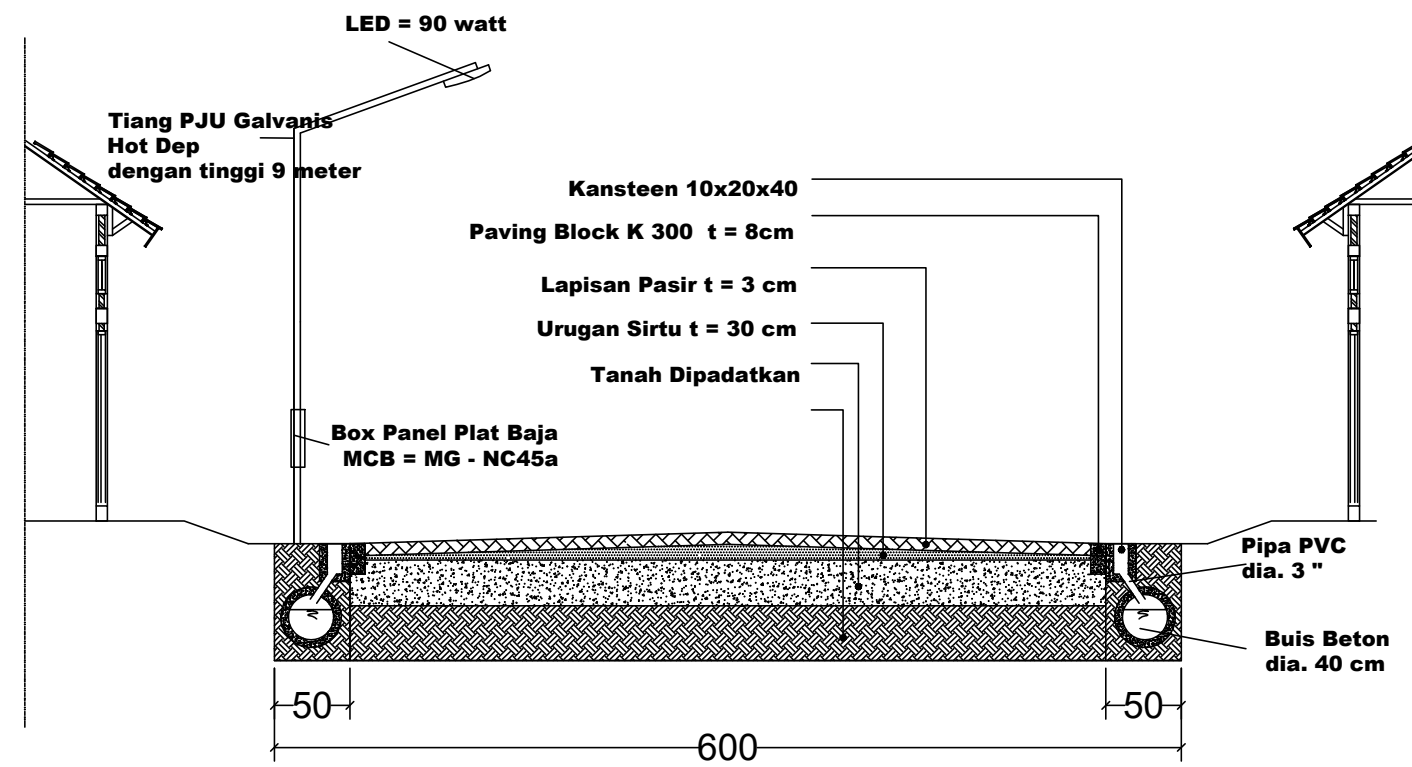
POTONGAN JALAN (ROW 6a)
