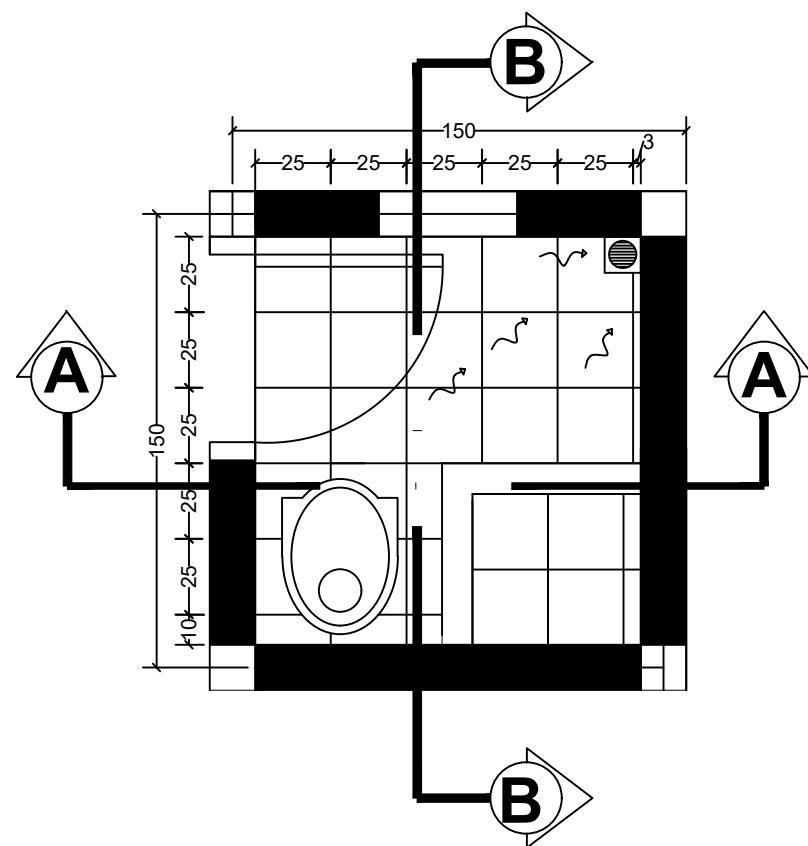
DETAIL KM/WC SKALA ; 1 : 25
