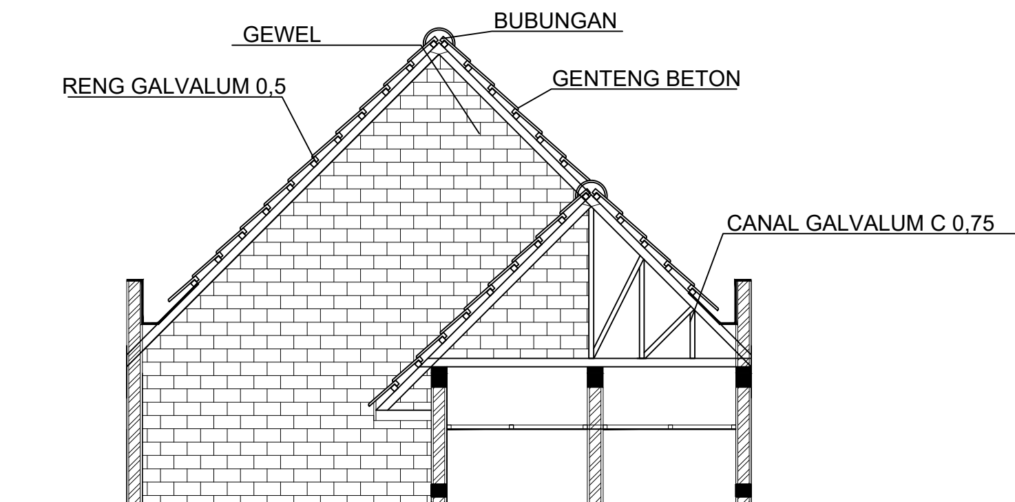
DETAIL POTONGAN KUDA KUDA BB SKALA ; 1 : 50
