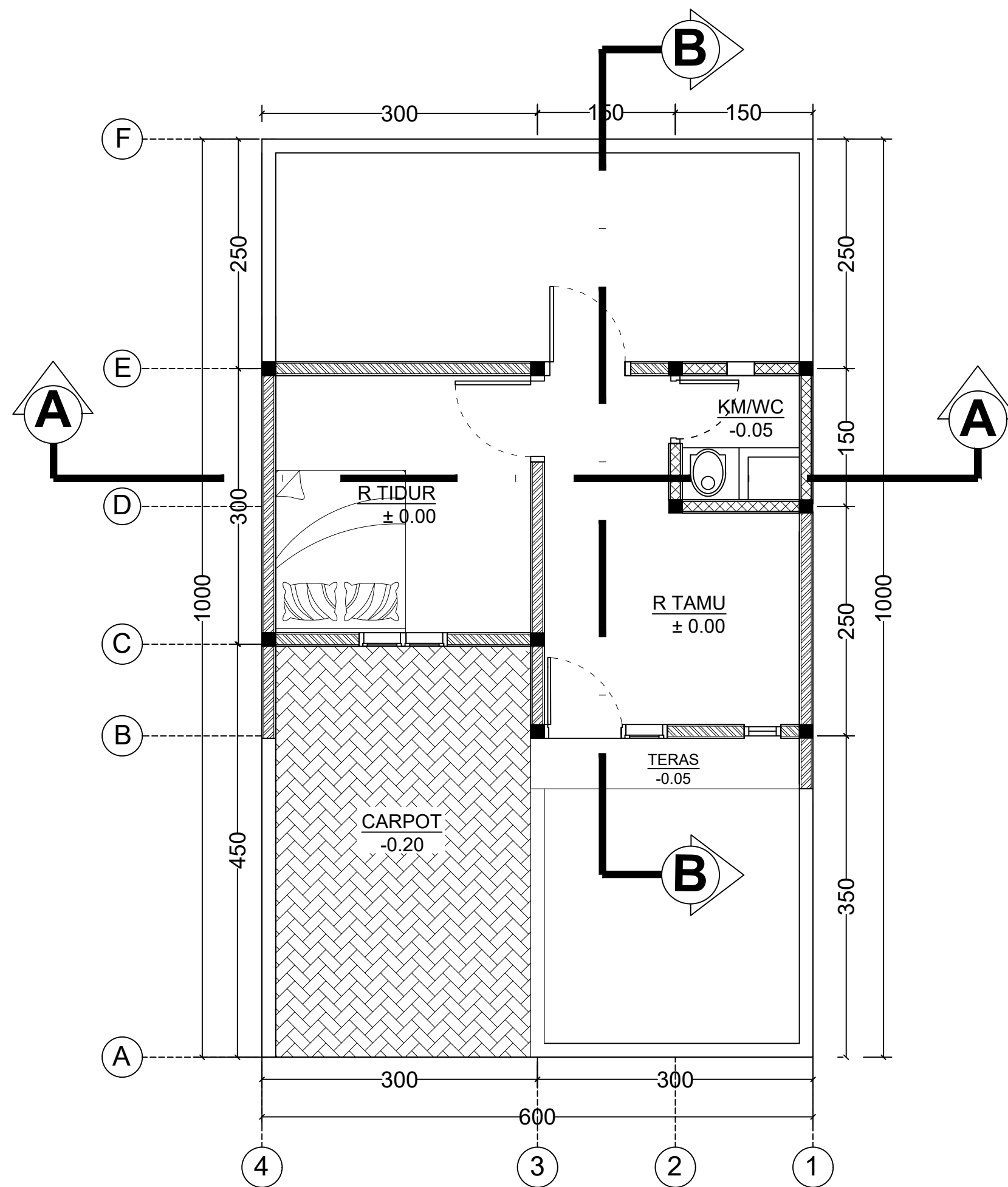
DENAH SKALA ; 1 : 50
