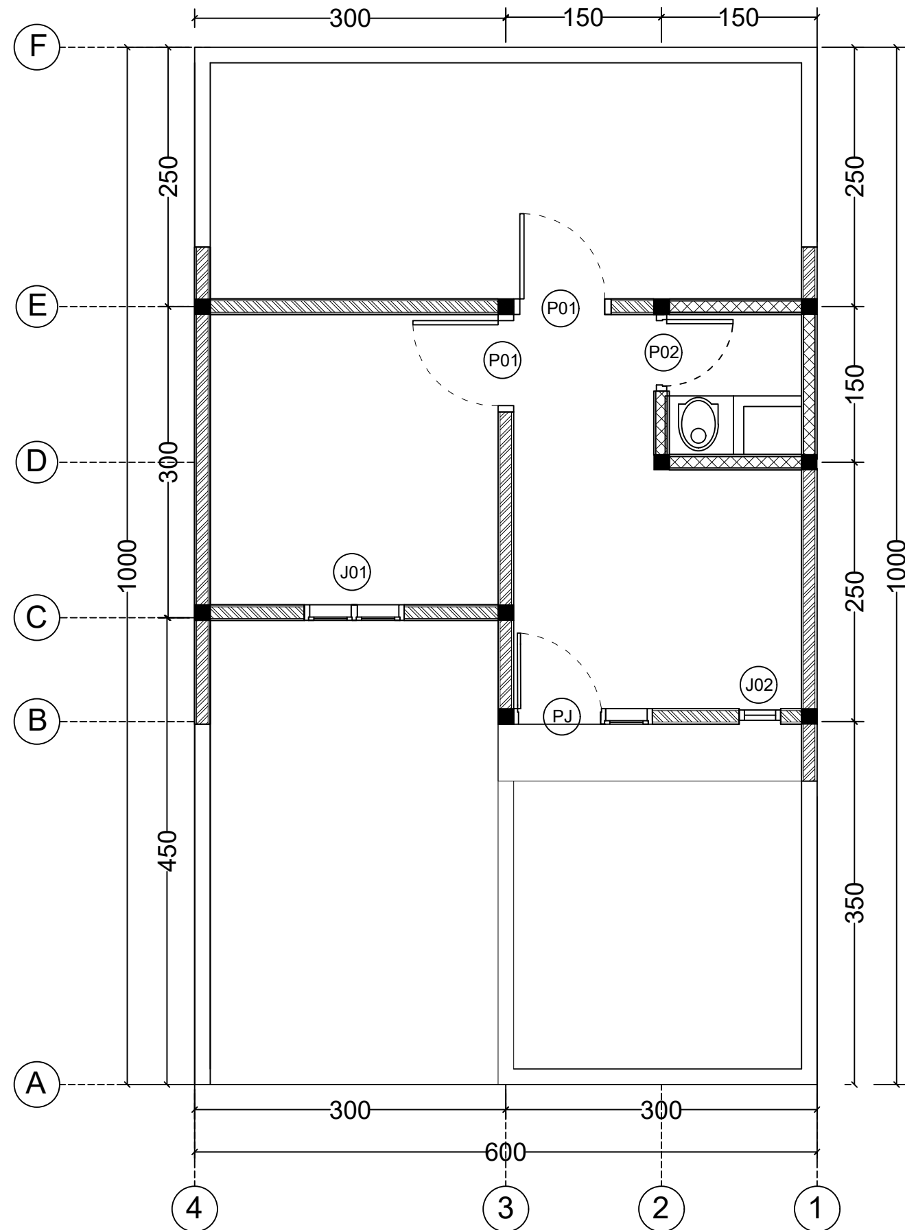
RENCANA KUSEN PINTU & JENDELA SKALA ; 1 : 50
