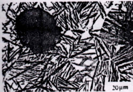
Gambar 4. Foto Bentuk mikrostruktur martensit adalah seperti jarum. Sumber : Bhadeshia, 2000
