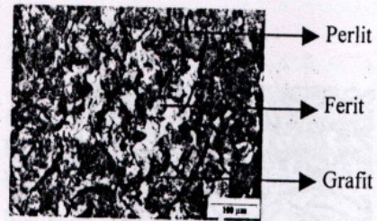
Gambar 3. Perlit (Bagian yang Gelap) dan Ferit (Bagian yang Terang), Etsa : Nital 2% Sumber : Bhadeshia, 2000
