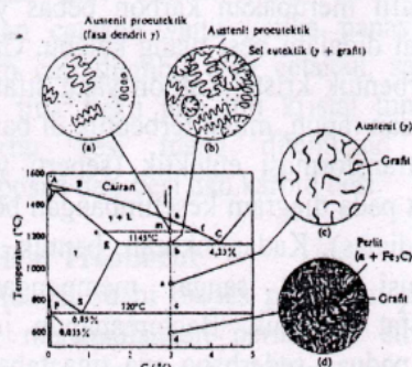
Gambar 2. Struktur Besi Tuang
