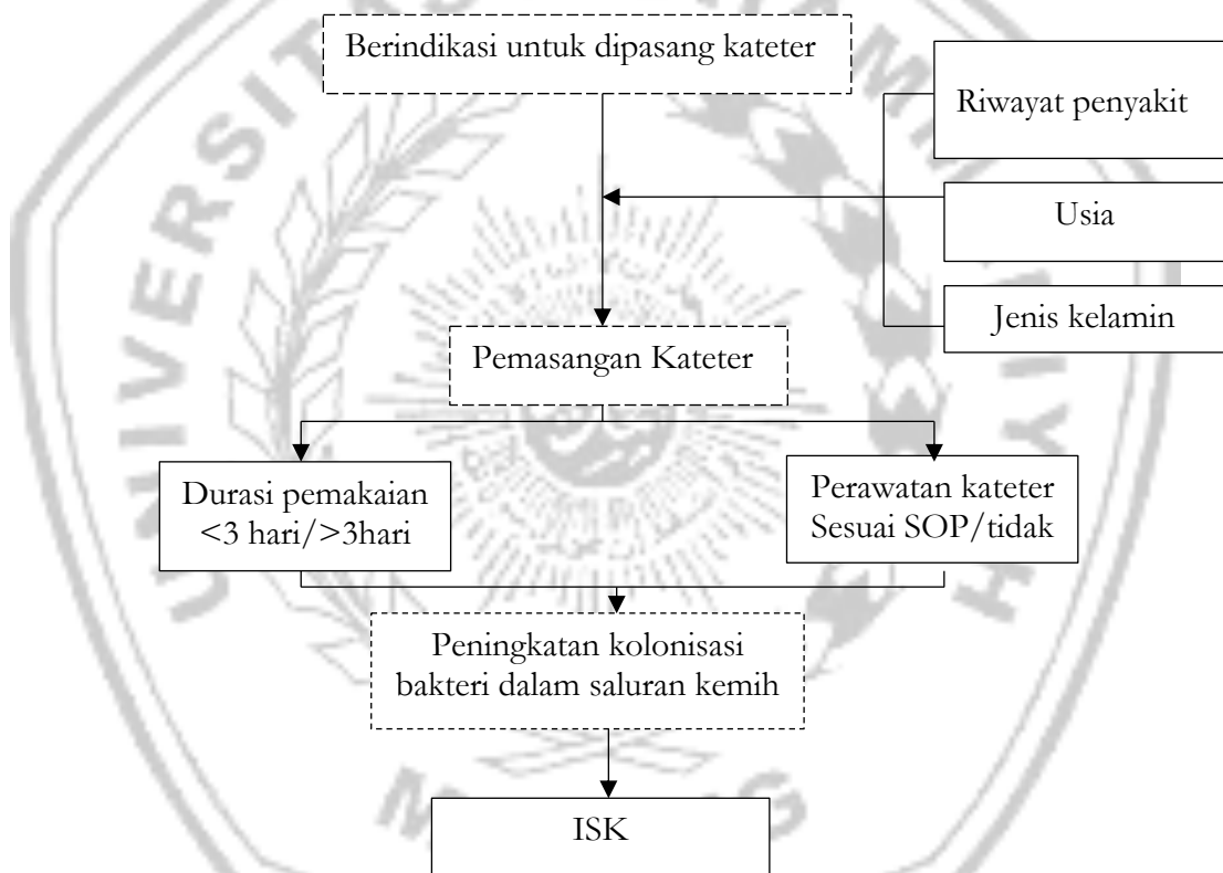
Gambar 3.1 Kerangka Konsep
