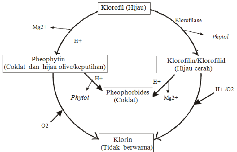
Gambar 10. Jalur degradasi klorofil
