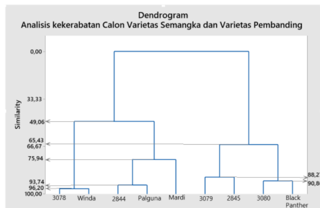
Gambar 5. Dendrogram Calon varietas semangka hibrida dan varietas pembanding berdasarkan semua parameter pengamatan.
