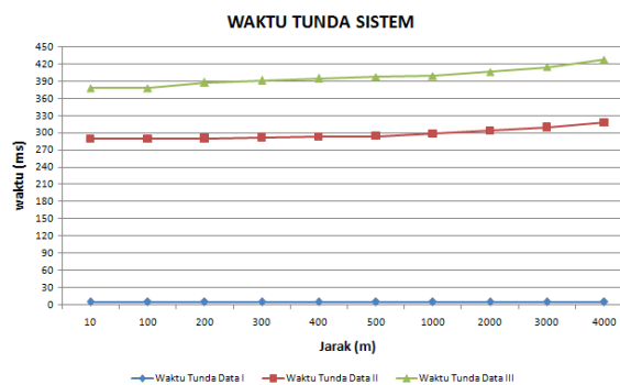
Gambar 15. Grafik Waktu Tunda Sistem
