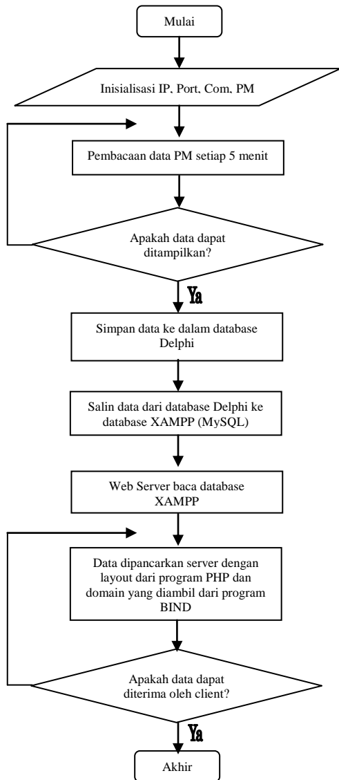
Gambar 4. Diagram Alur Pemrograman
