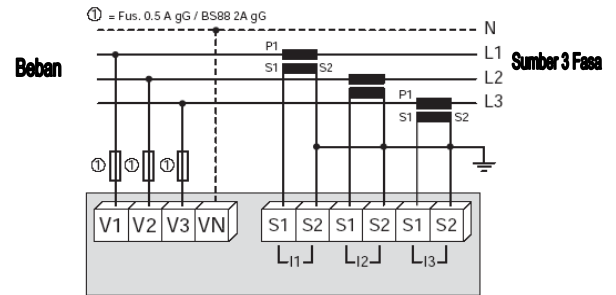
Gambar 3. Diagram pengawatan powermeter dengan beban dan sumber tegangan Komponen software yang digunakan dalam pembuatan alat ini antara lain:
