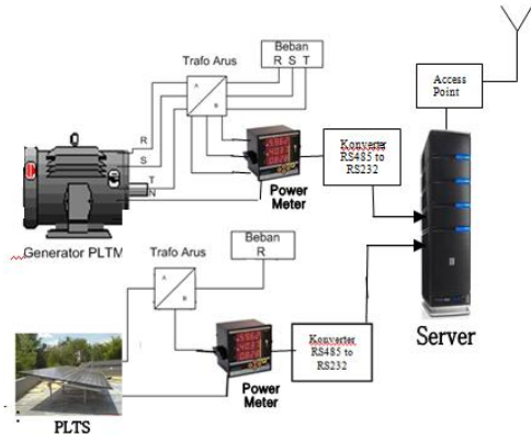
Gambar 1. Diagram Blok Alat
