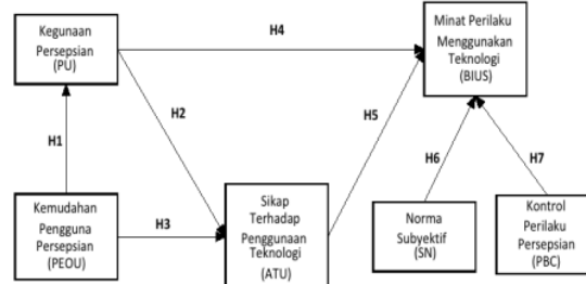
Gambar 1. Konstruk Penelitian
