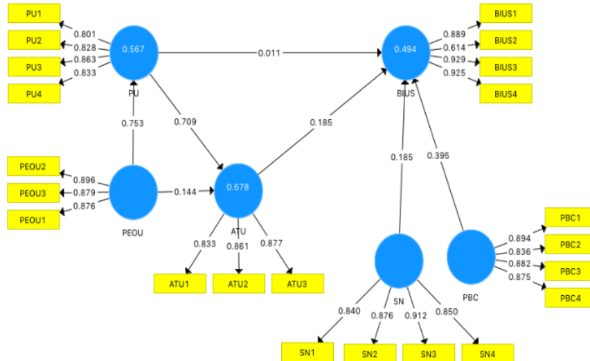
Gambar 4. Loading Faktor
