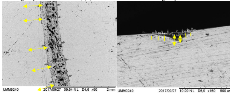
Gambar 7 Foto mikro permukaan baja ST41 dengan 100% pelumas mineral (a) lebar keausan dengan pembesaran 50×, (b) kedalaman keausan dengan pembesaran 150×
