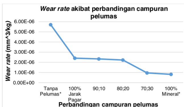
Gambar 8 Grafik hubungan laju keausan terhadap perbandingan campuran pelumas
