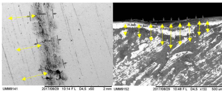
Gambar 4 Foto mikro permukaan baja ST41 dengan perbandingan pelumas 90:10 (a) lebar keausan dengan pembesaran 50 \times , (b) kedalaman keausan dengan pembesaran 150 \times
