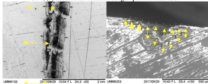
Gambar 3 Foto mikro permukaan baja ST41 dengan 100% minyak jarak pagar (a) lebar keausan dengan pembesaran 50 \times , (b) kedalaman keausan dengan pembesaran 150 \times
