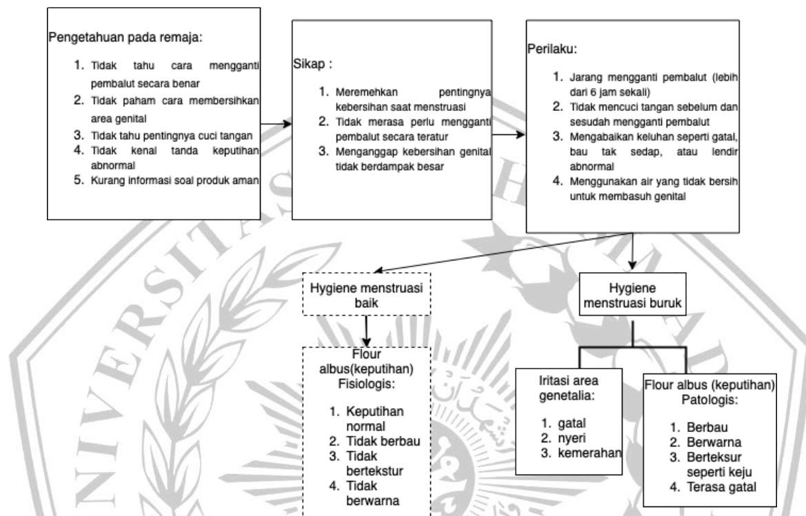
Gambar 3. 1 Lerangka Konseptual
