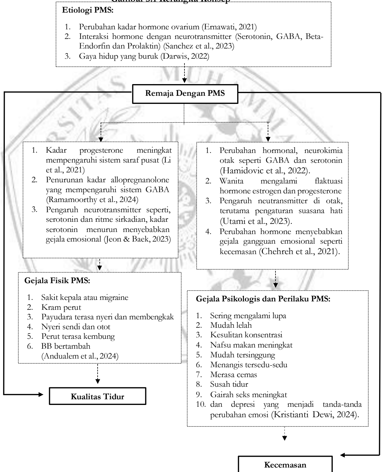
Gambar 3.1 Kerangka Konsep
