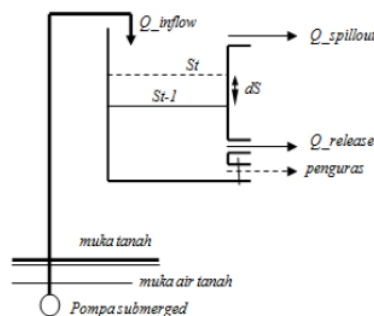
Gambar 2 Skema Keseimbangan Air Pada Tendon Penampung.
