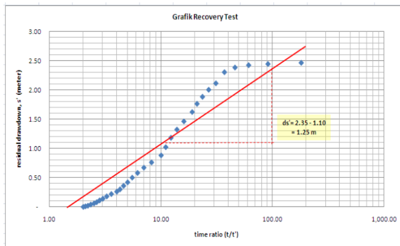
Gambar 8 Grafik Hubungan Waktu dan Residual Draw-down Kondisi Recovery
