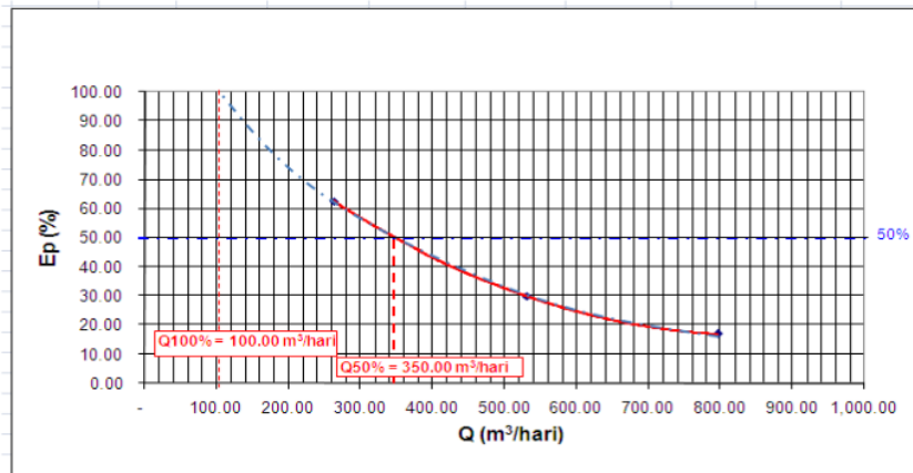
Gambar 11 Grafik hubungan debit (Q) dan efisiensi sumur (Ep)
