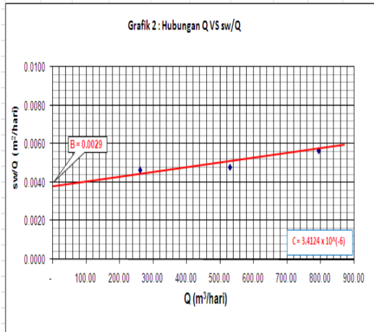
Gambar 10 Grafik hubungan debit (Q) dan Sw/Q
