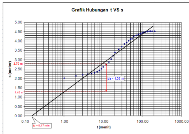
Gambar 7 Grafik hubungan waktu (t) dan draw-down (s) Metode Cooper-Jacop
