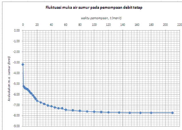
Gambar 3 Fluktuasi Muka Air Sumur Pada Uji Pompa Debit Tetap
