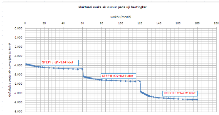
Gambar 5 Fluktuasi muka air sumur pada uji pompa bertingkat
