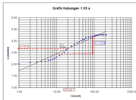
Gambar 6 Grafik hubungan waktu (t) dan draw-down (s) Metode Chow
