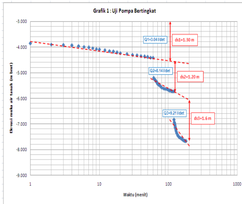
Gambar 9. Grafik hubungan waktu dan kedudukan m.a. sumur pada “step draw-down test”
