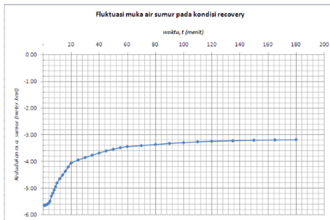
Gambar 4 Kenaikan Muka Air Sumur Pada Kondisi Recovery
