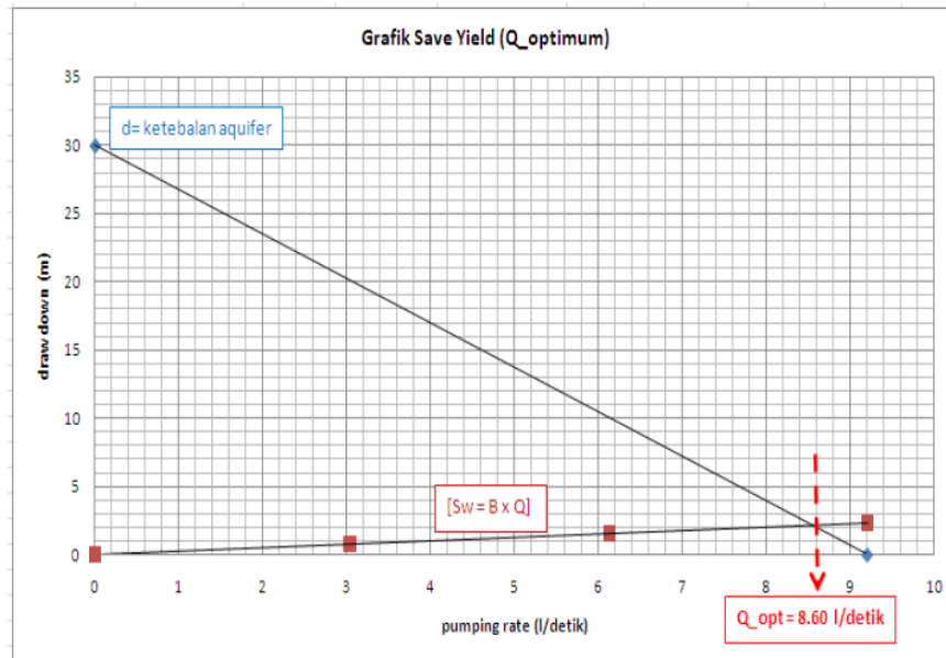
Gambar 13. Grafik save yield untuk menentukan Q optimum
