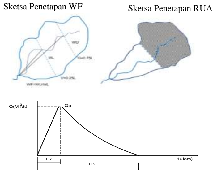
Gambar 1. Karakteristik HSS Gama I dan Sketsa Penetapan parameter WF dan RU (Sumber : Triatmodjo, 2008)
