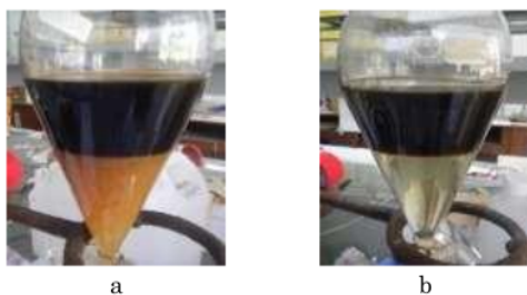
Gambar 1. Hasil Fraksinasi dengan Kloroform (a) Penambahan kloroform pertama kali dan (b) penambahan kloroform terakhir kali
