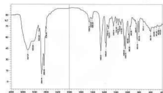
Gambar 8. Spektrum IR Isolat Murni
