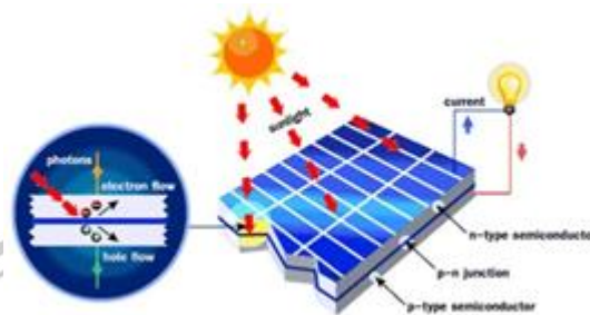
Gambar 2. 1 Cara bekerja sel surya silikon (Idris, 2020)
