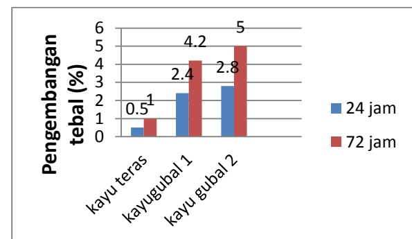
Gambar 5. Grafik rata-rata hasil uji pengembangan tebal.
