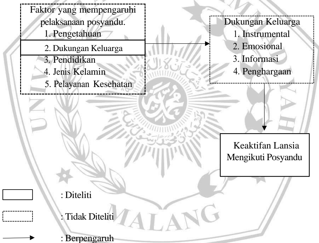
Gambar 3.1 Kerangka Konsep
