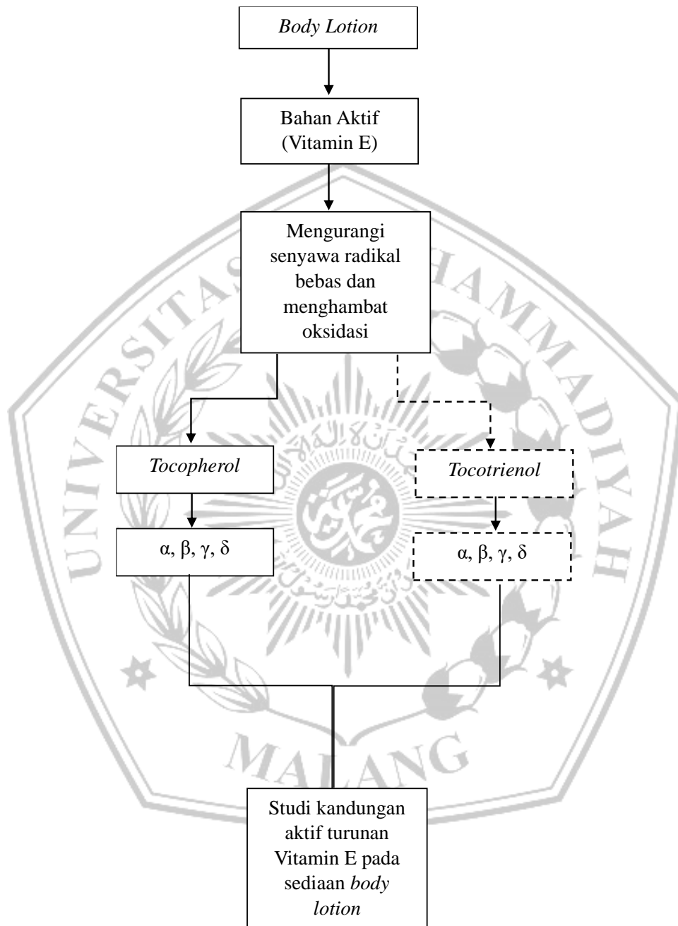
Gambar 3. 1 Kerangka Konseptual
