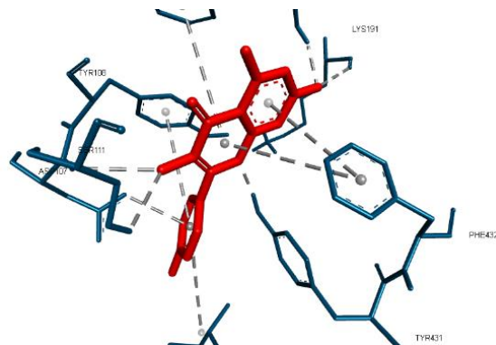
(b) Kaempferol
