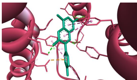
Pelargonidin
