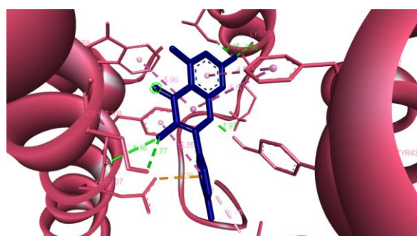
Kaempferol
