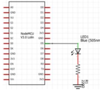
Gambar 6 Rangkaian Board NodeMCU V3 dengan LED
