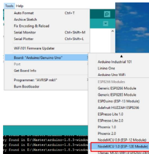
Gambar 5 Tampilan NodeMCU V3 Sudah Ada di Arduino IDE
