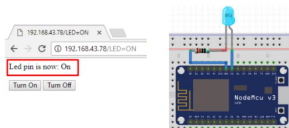
Gambar 10 Tampilan Kondisi LED Nyala
