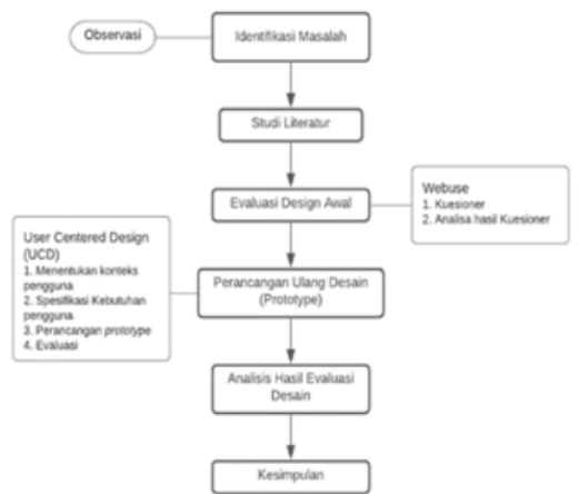
Gambar 3. Tahapan Penelitian
